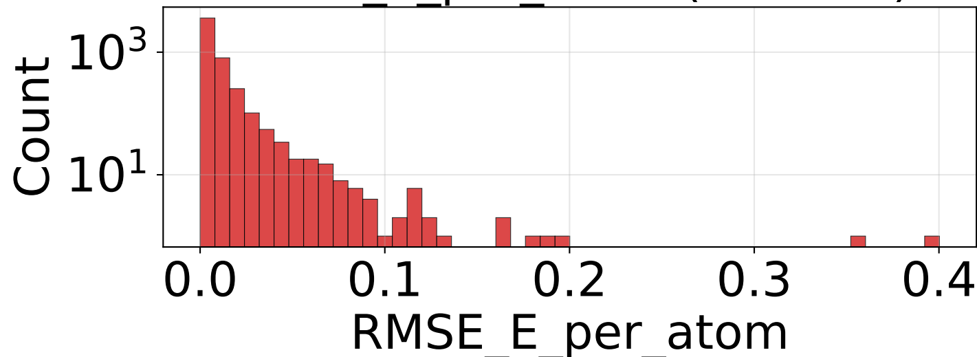
RMSE_E_per_atom (n=4950)
