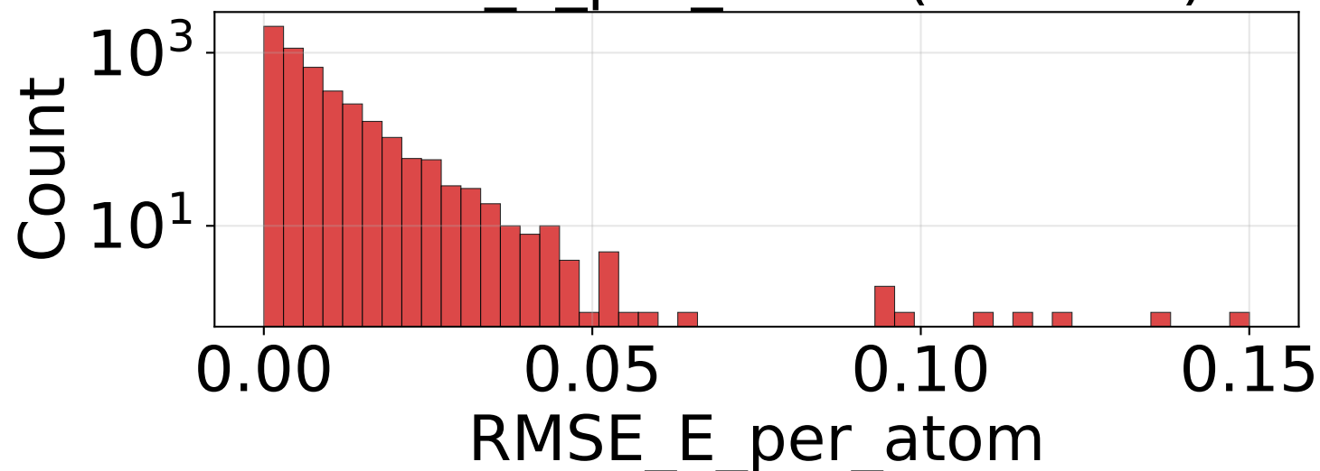
RMSE_E_per_atom (n=4950)
