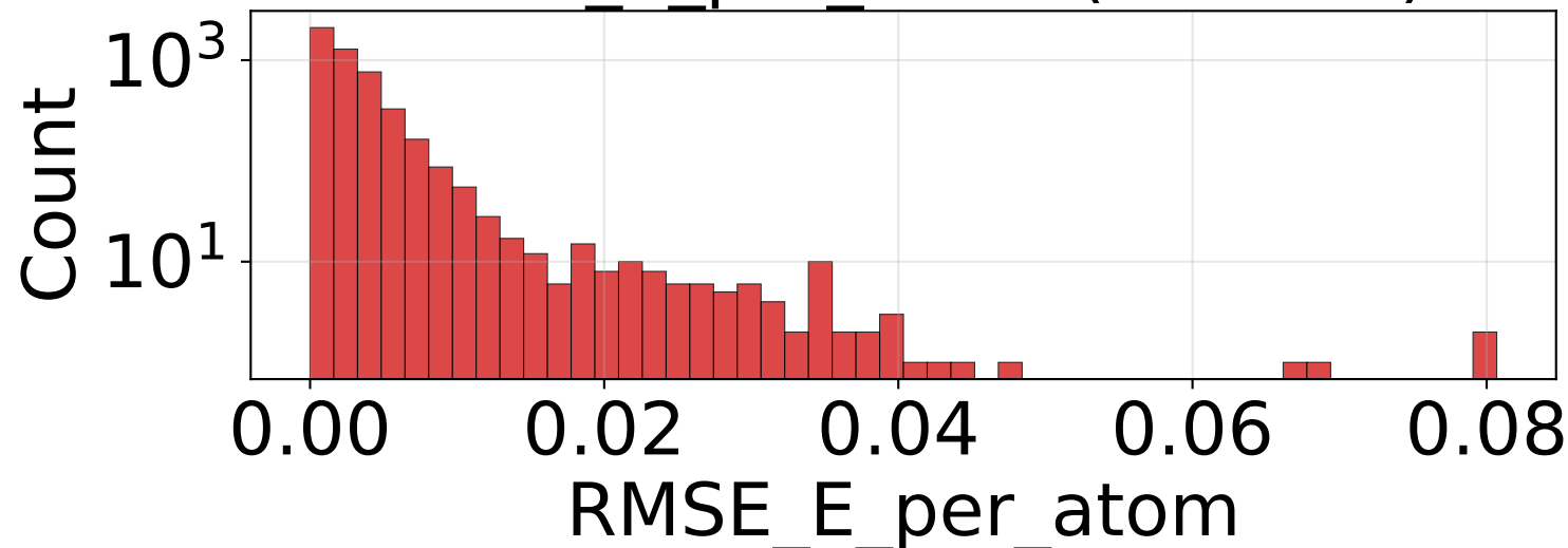
RMSE_E_per_atom (n=4950)
