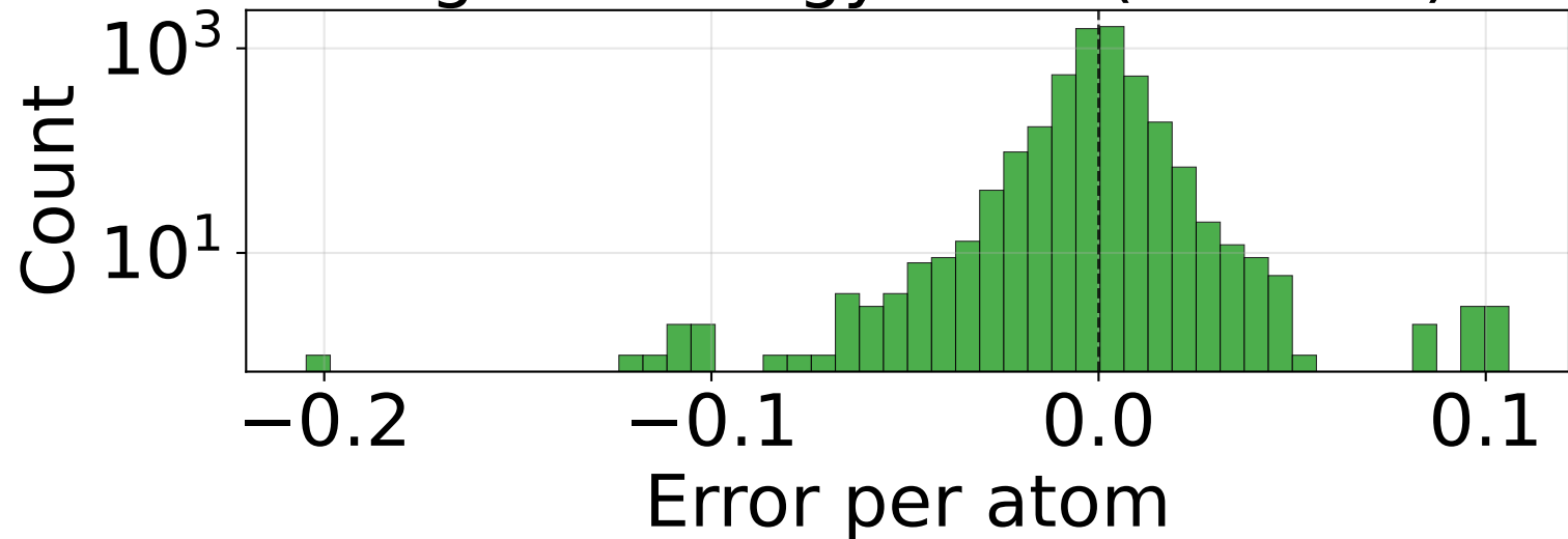
RMSE_E_per_atom (n=4950)
