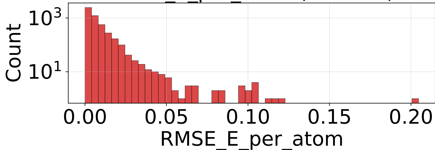
RMSE_E_per_atom (n=4950)
