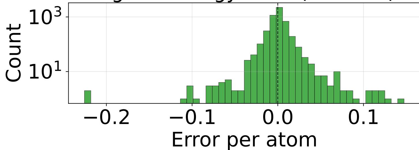
RMSE E_per_atom (n=4950)
