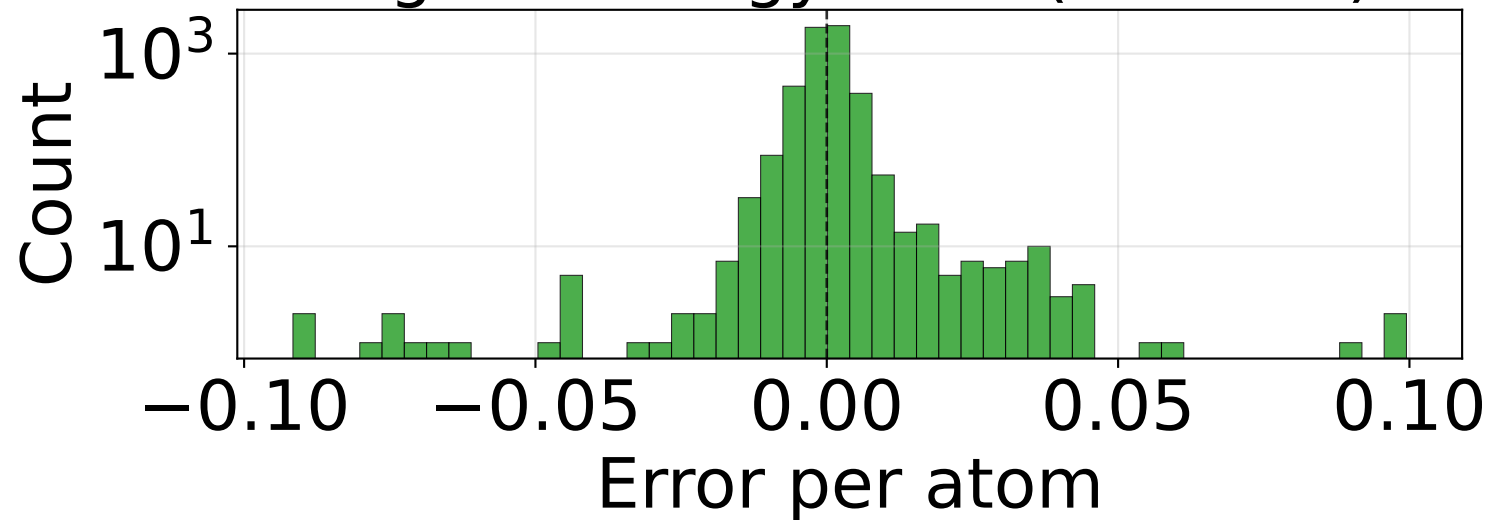
RMSE_E_per_atom (n=4950)
