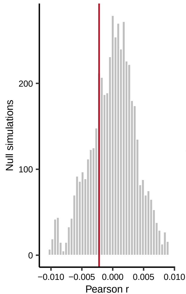
Circular-shift null
