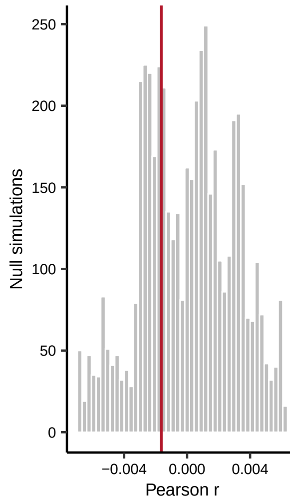
Circular-shift null
