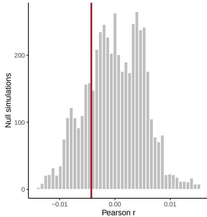
Circular-shift null
