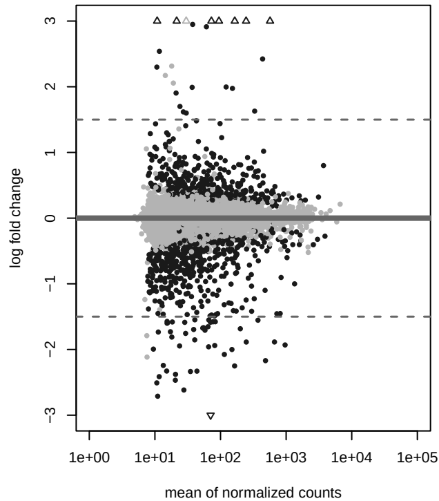
GOA_TC apeglm
