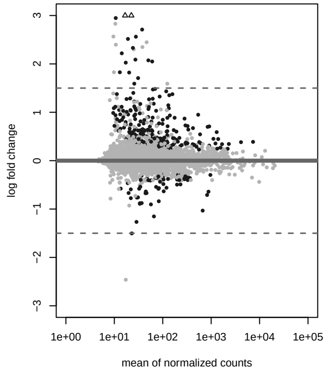
FOW_TC apeglm
