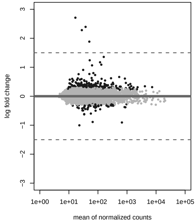
FOW_TC ashr
