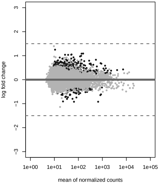
FOW_TC normal
