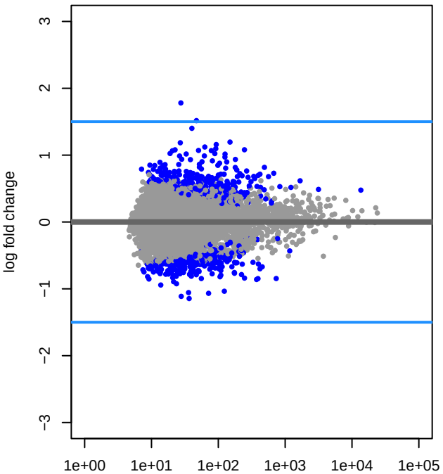
FDO_TC normal
