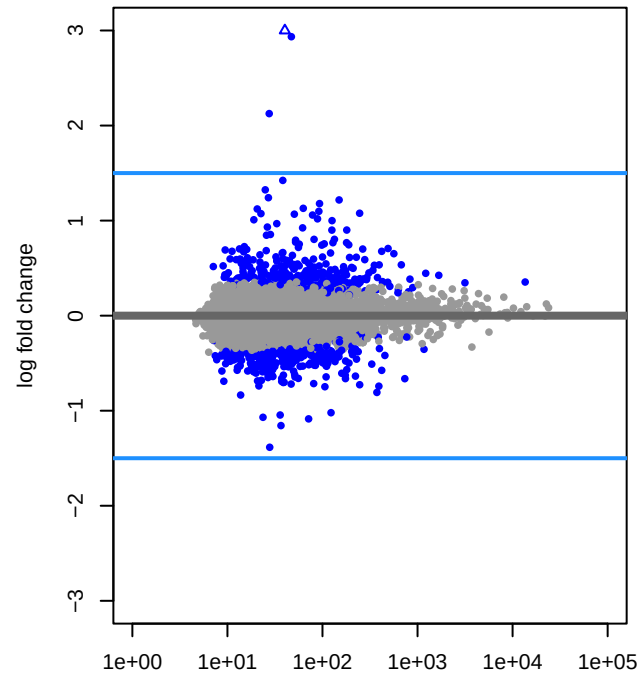
FDO_TC ashr
