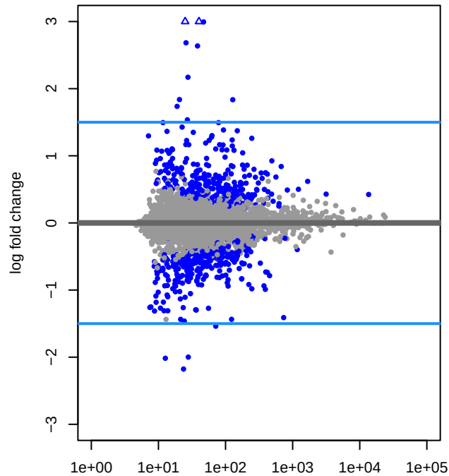
FDO_TC apeglm
