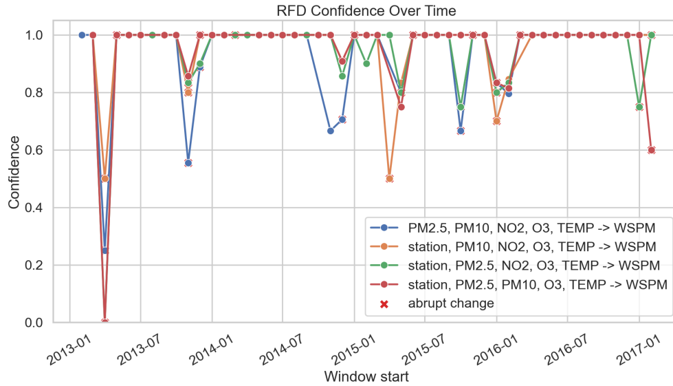
Figura 3: Continuous profiling mensile delle RFD scoperte da DiMe.
