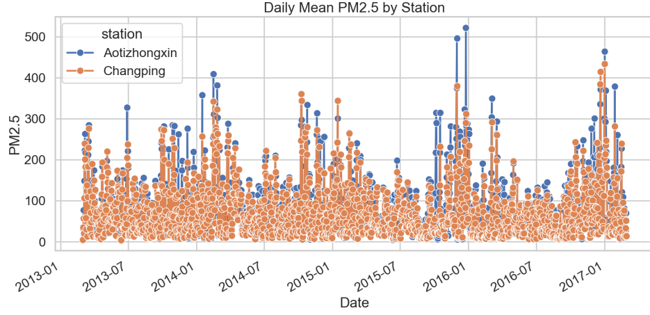
Figura 1: Media giornaliera di PM2.5 per stazione.
