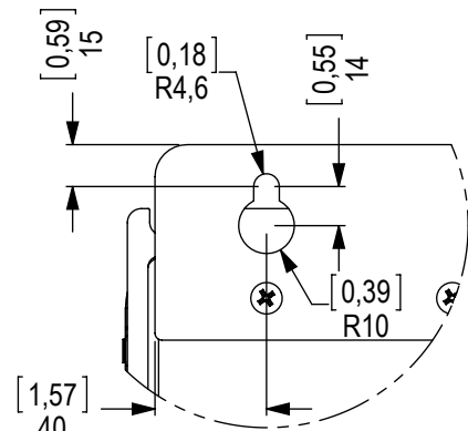
DETALHE A ESCALA 1 : 3
