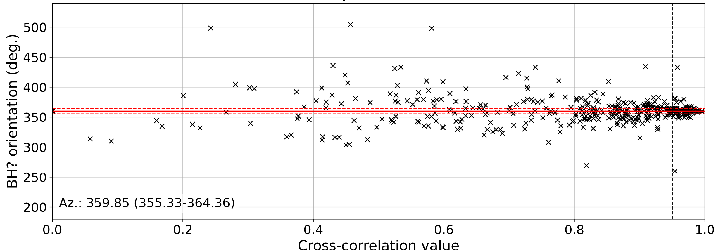
DLOPy result BK.LGMB
