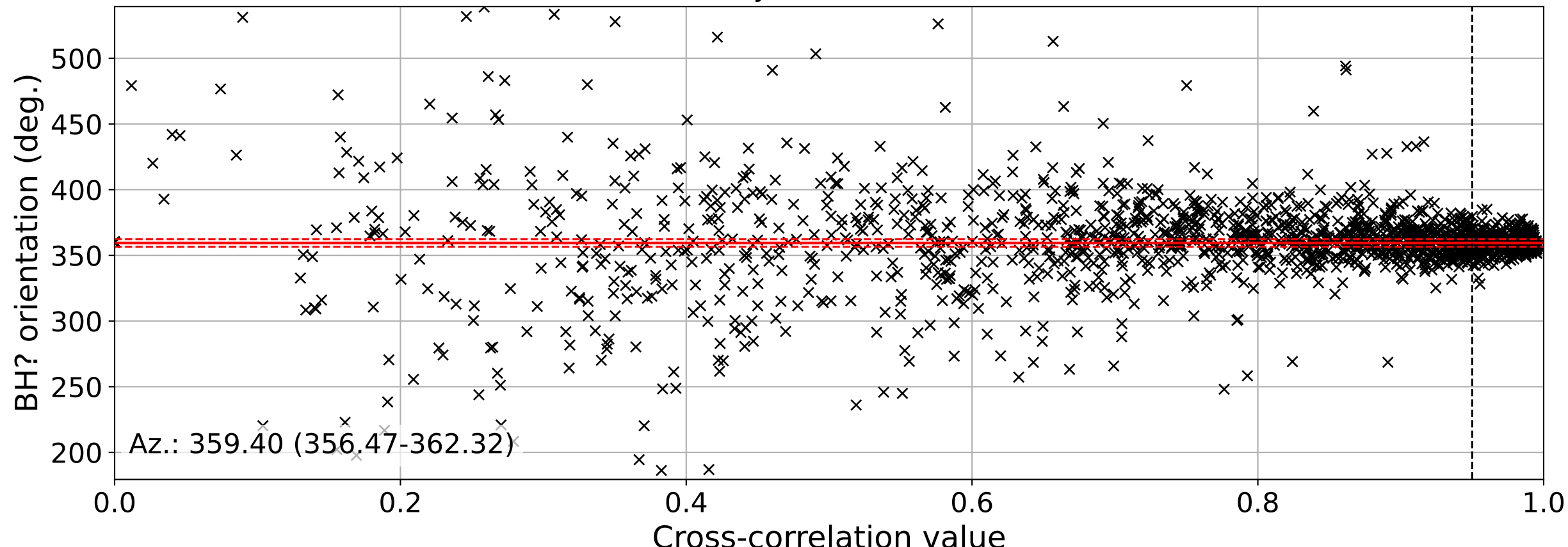
DLOPy result BK.PACP
