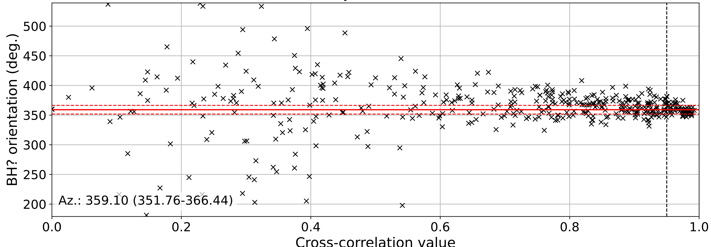
DLOPy result BK.LSIB
