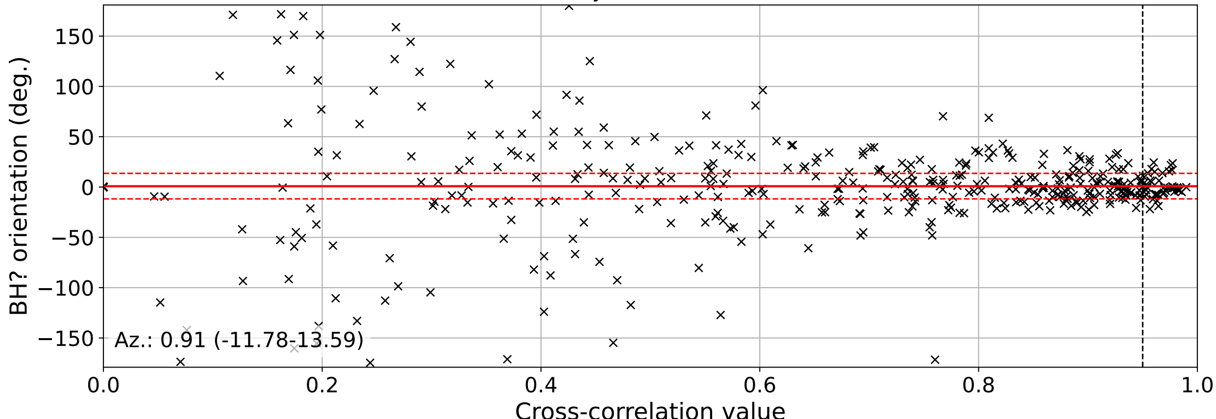
DLOPy result BK.TULE
