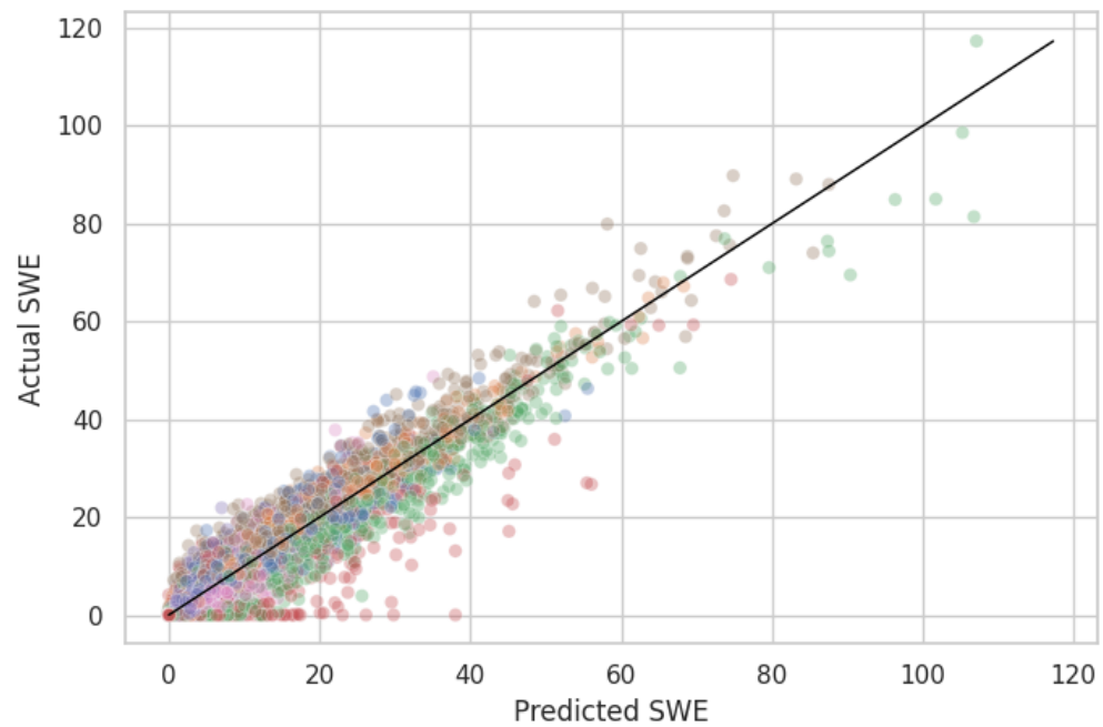
Predicted vs Actual SWE
