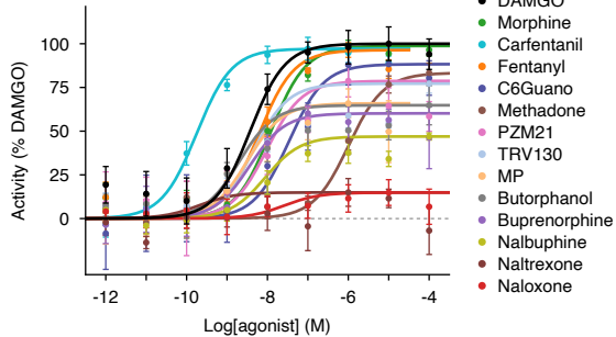
TRUPATH GI1 BRET assay
