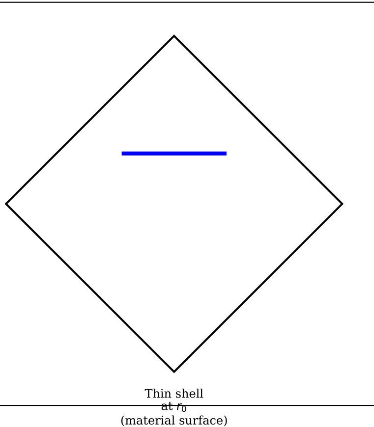
Gravastar
