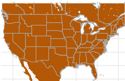
ssp245
