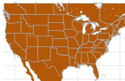
ssp585
