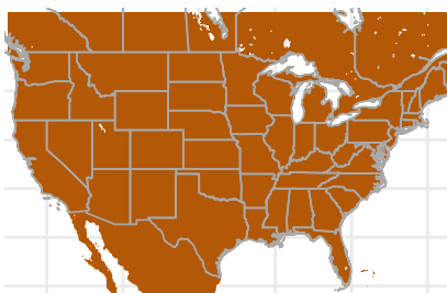
ssp370
