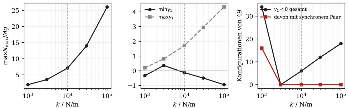
Abbildungung 9.6: Kennzahlen gegen die Kontaktsteifigkeit. Links die maximale Spitzenkraft, Mitte die Spannweite der Schiefe, rechts die Zahl der Konfigurationen mit negativer Schiefe und davon jene mit synchronem Modulpaar. Punktiert der Basisparametersatz.
