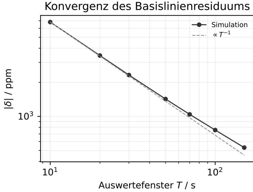
Abbildung 9.1: Doppeltlogarithmische Darstellung des Residuums gegen die Fensterlänge. Der angepasste Exponent beträgt -0,945 ; die gestrichelte Gerade zeigt \propto T_w^{-1} . Die Achsenbeschriftung T entspricht T_w .
