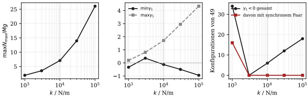
Abbildung 9.6: Kennzahlen gegen die Kontaktsteifigkeit. Links die maximale Spitzenkraft, Mitte die Spannweite der Schiefe, rechts die Zahl der Konfigurationen mit negativer Schiefe und davon jene mit synchronem Modulpaar. Punktiert der Basisparametersatz.
