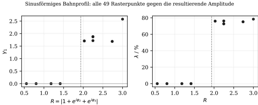
Abbildung 9.5: Alle 49 Rasterpunkte des Sinus-Sweeps gegen R . Links die Schiefe, rechts der Liftoff-Anteil. Gestrichelt die quasistatische Schwelle R_c^{\text{qs}} = 1,94 ; die tatsächliche Schwelle liegt nach Gleichung (9.7) bei 1,45.
