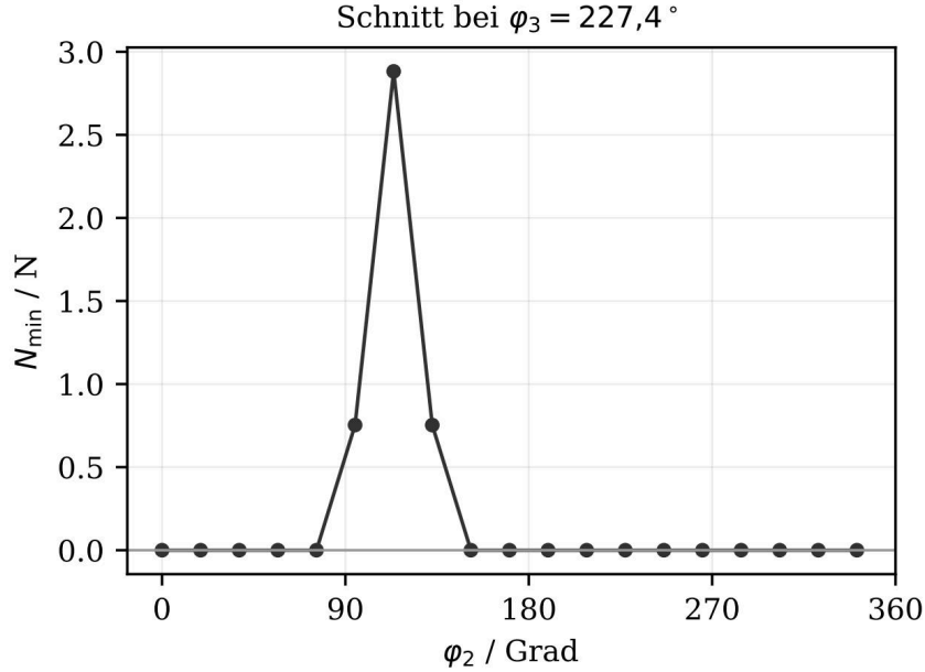
Abbildungung 9.4: Minimale Kontaktkraft entlang \varphi_2 bei festem \varphi_3 = 227,4^\circ . Drei der neunzehn Rasterpunkte dieses Schnitts sind liftoff-frei. Die Rasterweite von 18,9^\circ löst den Verlauf zwischen ihnen nicht auf.
