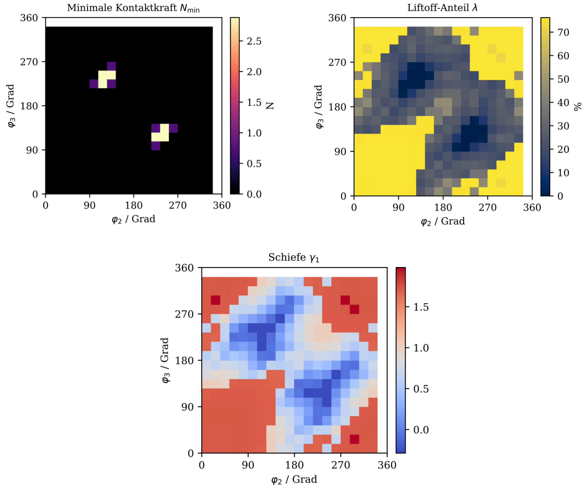
Abbildung 9.3: Zielfunktionale über dem Raster der relativen Phasenkonfigurationen. Oben links die minimale Kontaktkraft N_{\min} , oben rechts der Liftoff-Anteil \lambda , unten die Schiefe \gamma_1 . Die drei Karten zeigen dieselbe Struktur aus verschiedenen Blickwinkeln: Der Bereich mit N_{\min} > 0 ist genau der Bereich mit \lambda = 0 .
