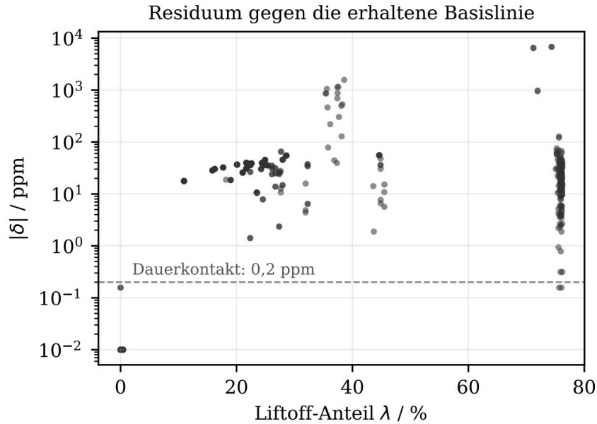
Abbildung 9.2: Betrag des relativen Residuums |\delta| nach Gleichung (9.2) gegen den Liftoff-Anteil, für alle 361 Konfigurationen des Archivlaufs (Burn-in fest 5 s). Logarithmische Ordinate. Bei Dauerkontakt liegt das Residuum am numerischen Boden der Integration; mit wachsender Intermittenz steigt es um vier Größenordnungen.
