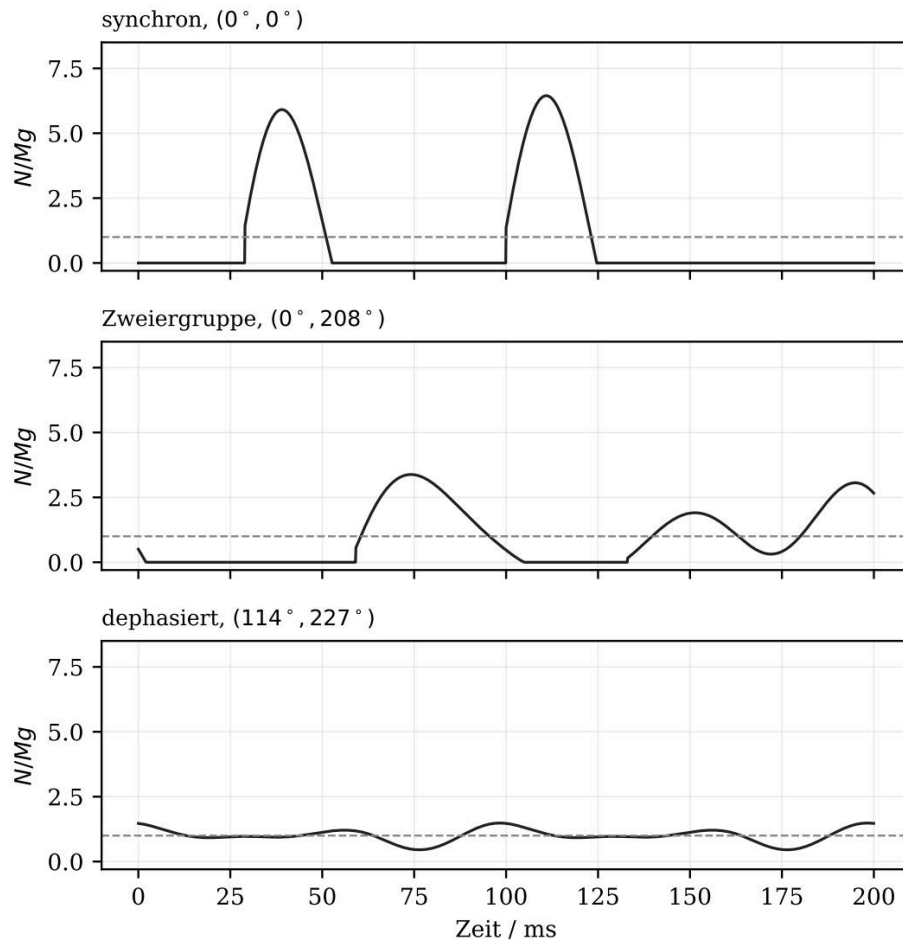
Abbildung 6.1: Simulierter Kraftverlauf über zwei Anregungsperioden für drei Regime, normiert auf die Basislinie. Gestrichelt: N = Mg . Oben und Mitte heben ab, unten bleibt der Kontakt erhalten.
