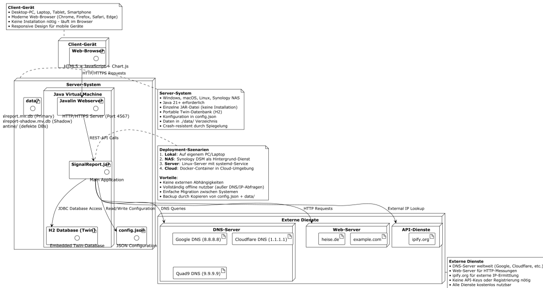
Abbildung 13: Vollständiges Deployment-Diagramm
