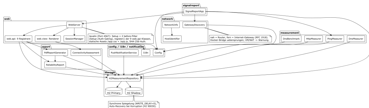
Abbildung 9: Vollständiges Komponenten-Diagramm
