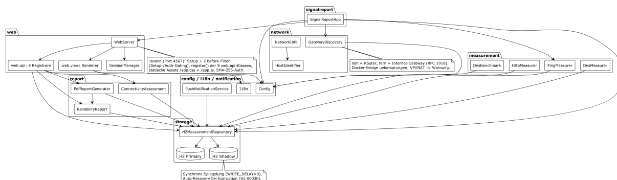
Abbildung 2: Komponenten-Übersicht von SignalReport
