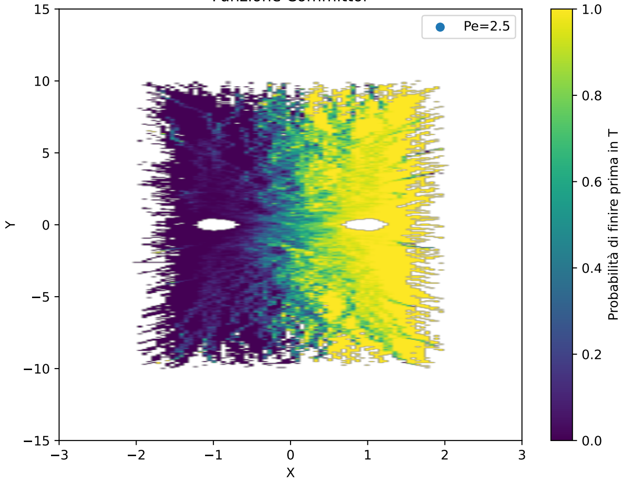
Funzione Committor
