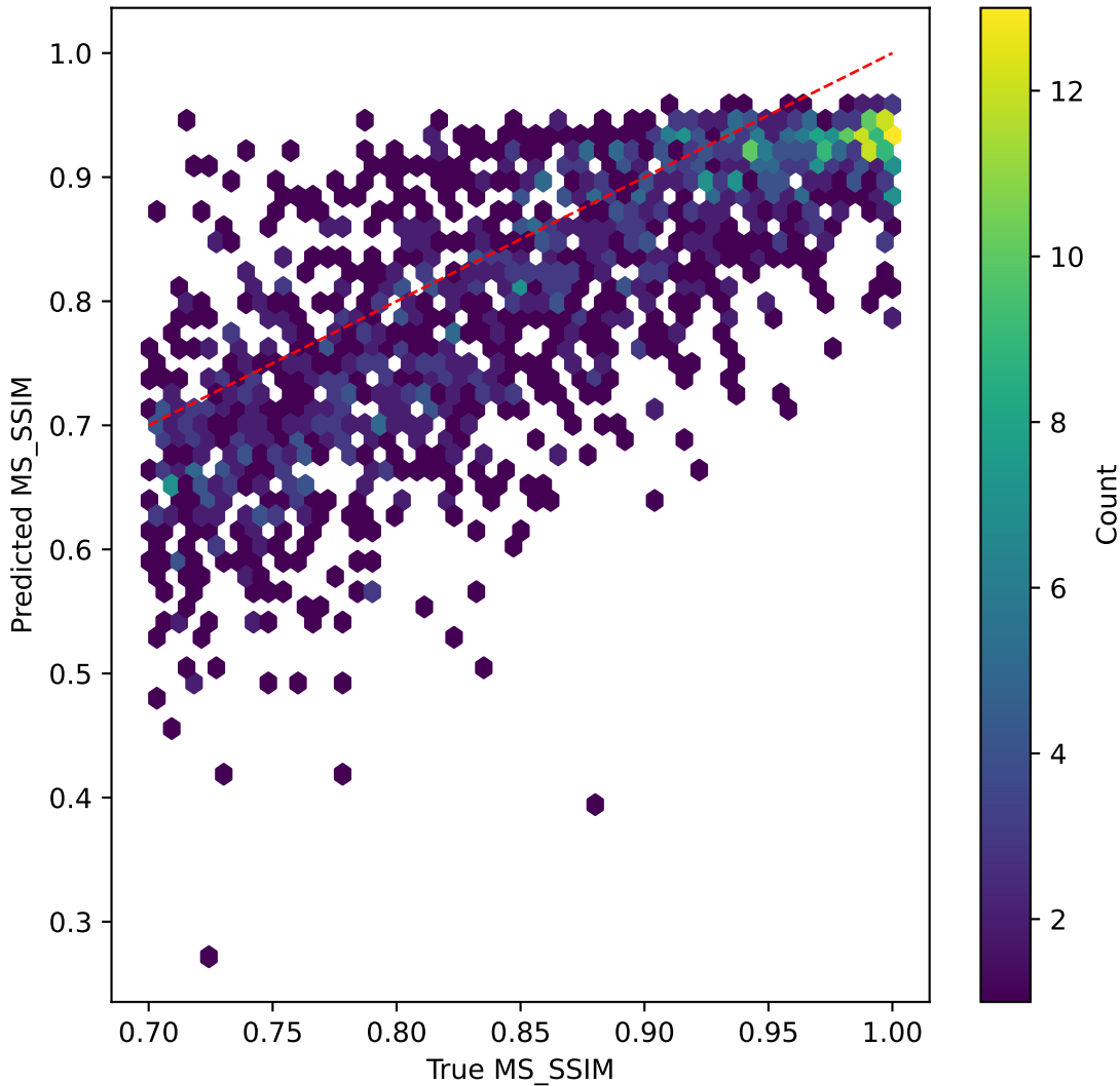
tinyvit on MS_SSIM | R^2=-0.000
