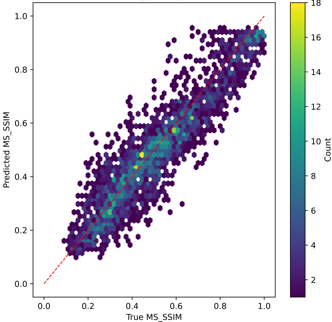
tinyvit on MS_SSIM | R^2=0.844
