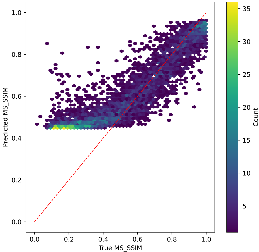
vit on MS_SSIM | R^2=0.595
