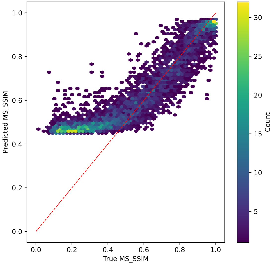
tinyvit on MS_SSIM | R^2=0.607
