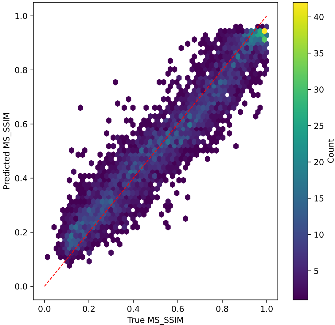
tinyvit on MS_SSIM | R^2=0.849
