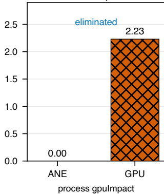
GPU impact
