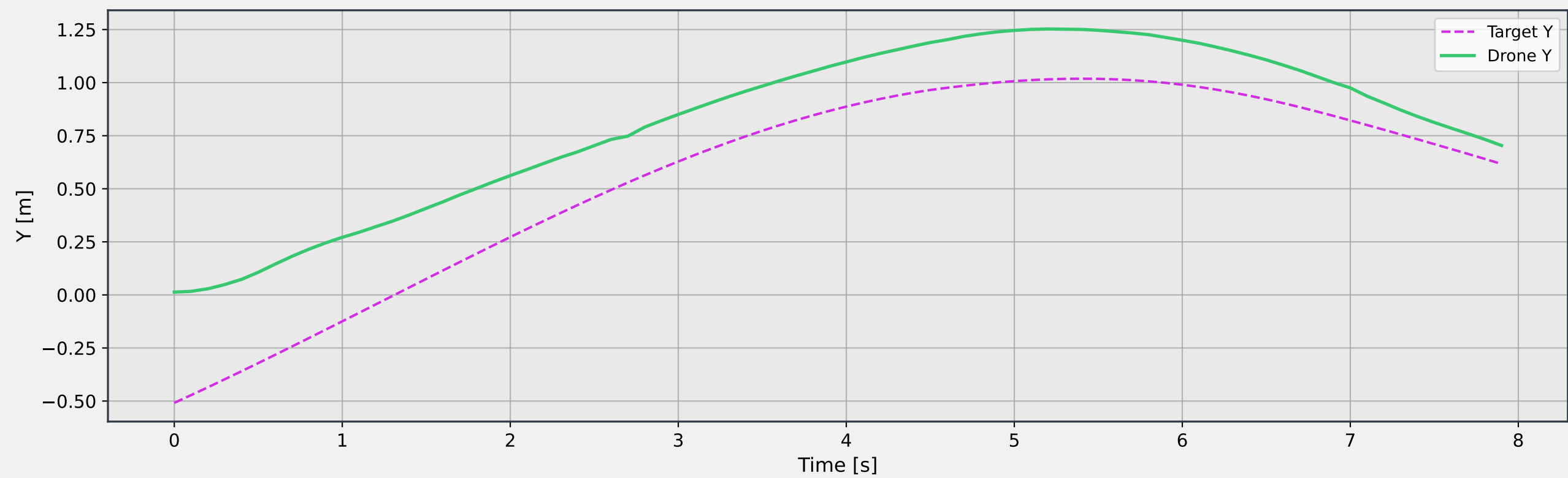
Y Tracking
