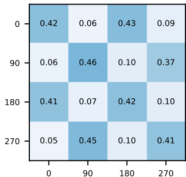
digit 6: 0.109
