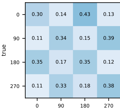
digit 5: 0.366
