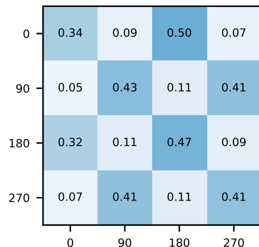
digit 8: 0.415
