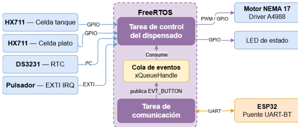
FIGURA 3.11. Diagrama de integración hardware-software del sistema.
