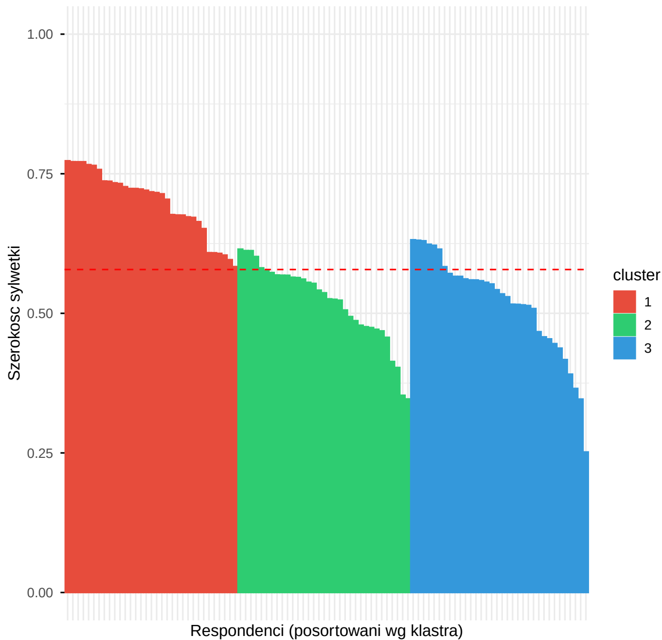
Wykres sylwetki dla k = 3 skupien
