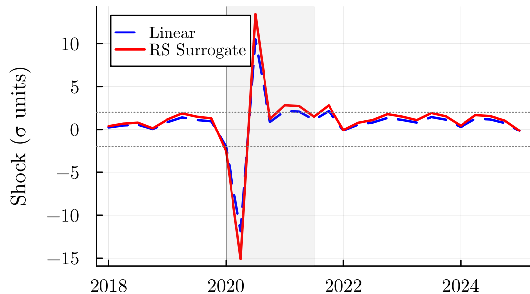
TFP ( \varepsilon_{\pi} )
