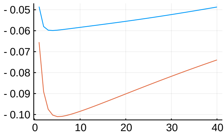
r^*
