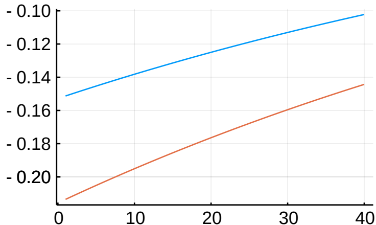
r^*
