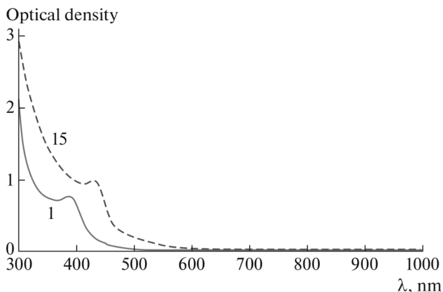
Рис. 2.4. Спектры оптической плотности КТ CdSe, полученных в поточном синтезе при различном времени роста (1 и 15 мин.) [86]
