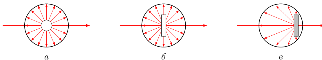
Рис. 2.19. Схемы измерений индикатрис рассеяния света: а) коллоидный раствор, слой на прозрачной (б) и отражающей (в) подложках [101]
