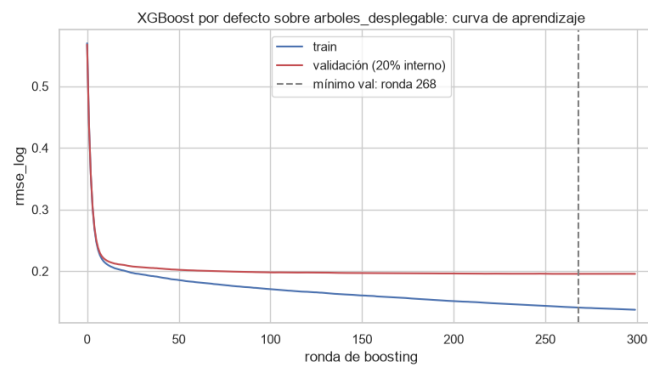
Figura 3. Curva de aprendizaje de XGBoost con hiperparámetros por defecto sobre la variante desplegable, con un 20 % del entrenamiento reservado para validación. Fuente: cuaderno 06.
