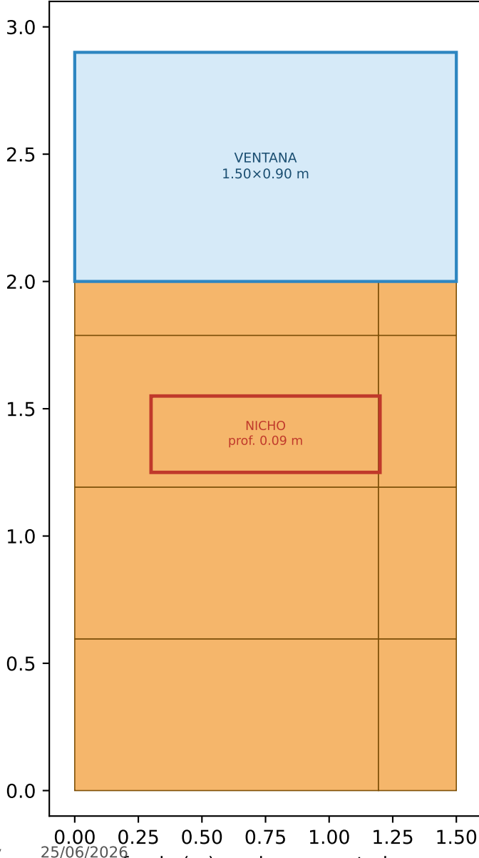
Regadera 3 (P.A.)
