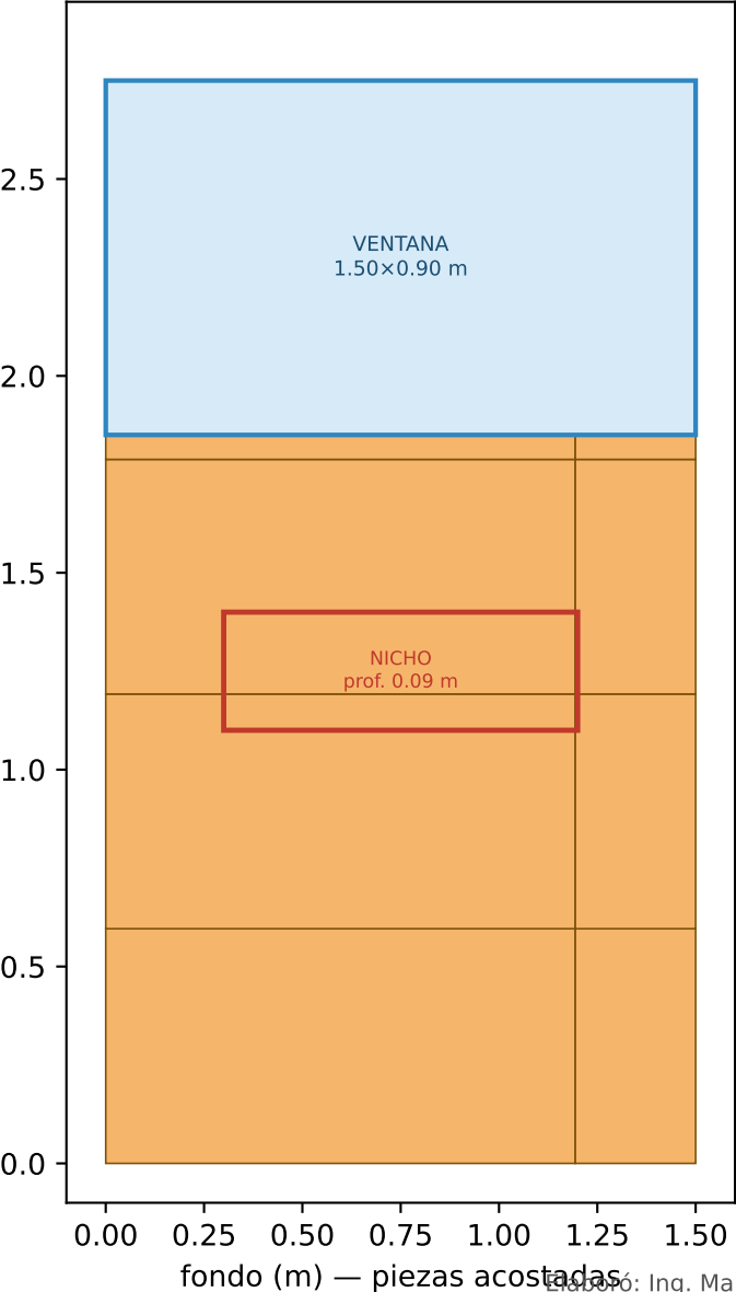
Regadera 1 (P.B.)
