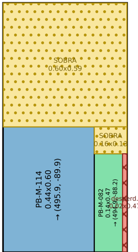
Baldosa M-51 · 2 pza(s)
