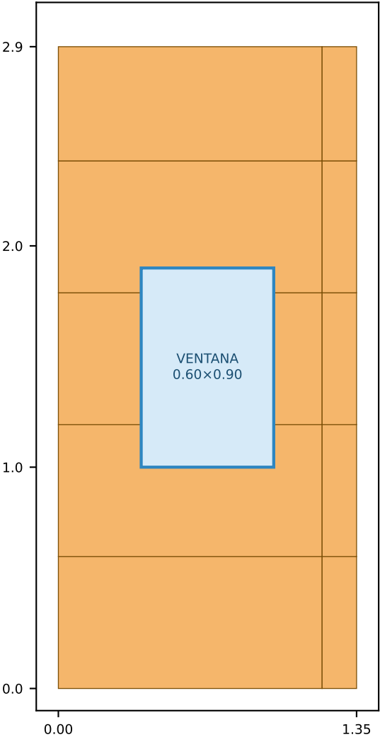
Regadera 1 (P.A.) muro fondo 1.35 × 2.90 m 3 caras – ventana = 10.77 m²
