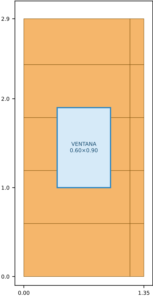
Regadera 2 (P.A.) muro fondo 1.35 × 2.90 m 3 caras – ventana = 10.77 m²
