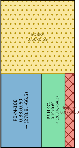
Pieza M-81 · 2 recorte(s)
