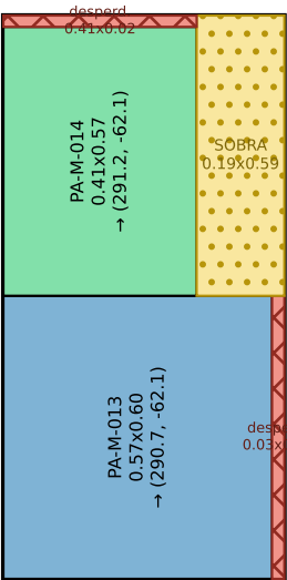
Pieza M-61 · 2 recorte(s)
