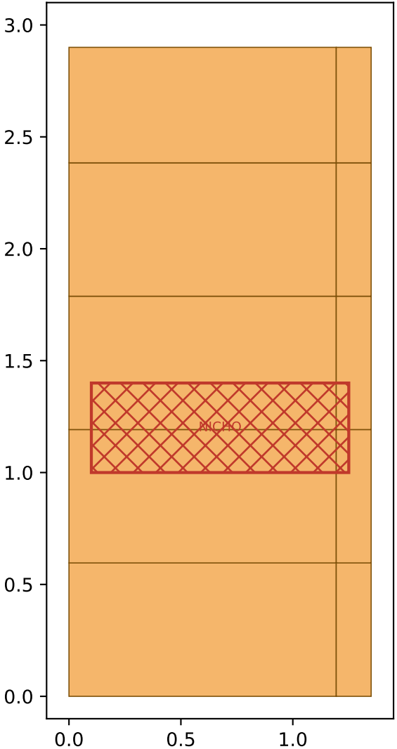
Regadera 3 (P.A.) muro fondo 1.35×2.90 m · 3 caras=11.31 m²
