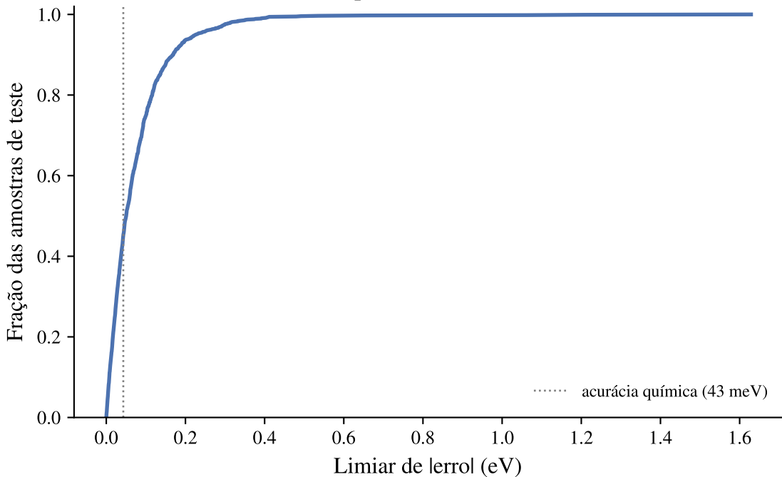
etr_emb_pca99 - cumulative error
