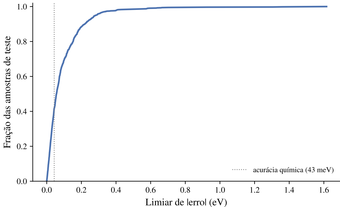
etr_baseline - cumulative error
