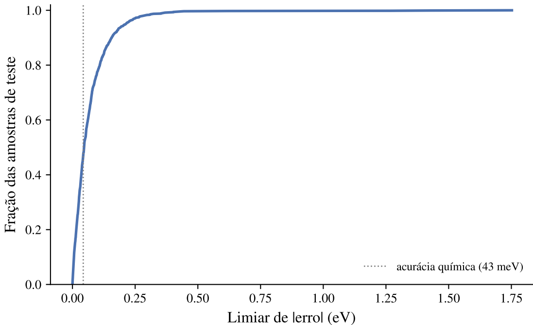
etr_emb_all - cumulative error
