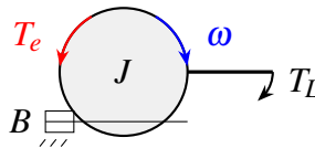
Figura 1 – Corpo livre do rotor
