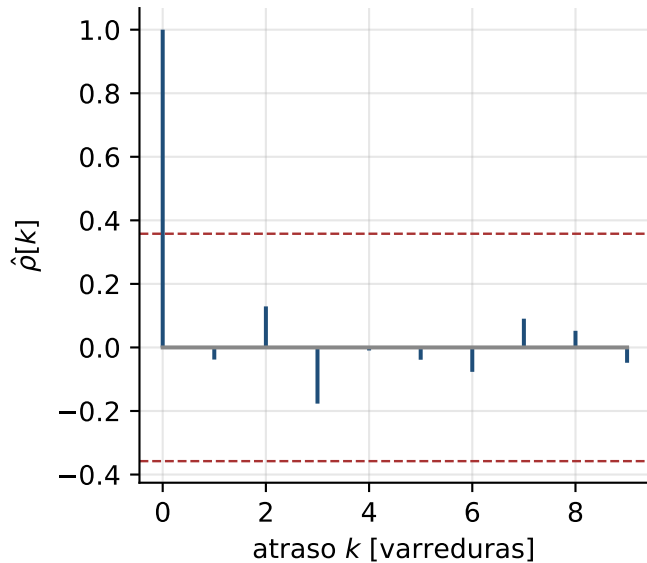
(b) autocorrelação (repouso)
