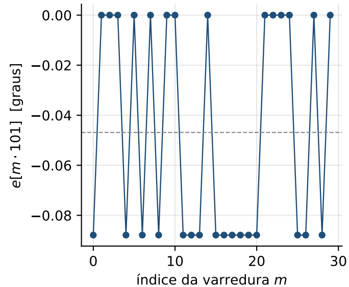
(a) repouso, 30 realizações
