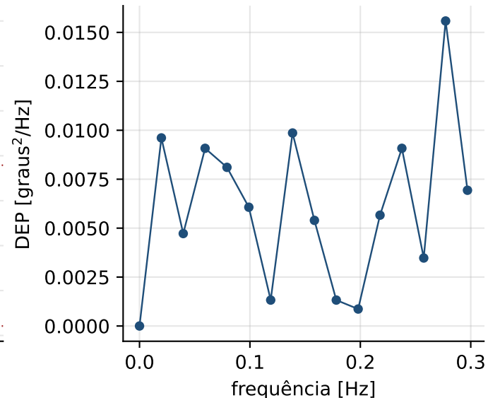
(c) periodograma (repouso)
