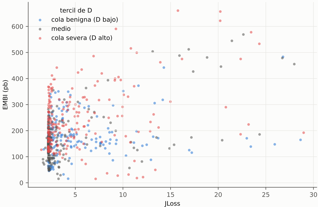
Complementariedad: dispersión JLoss vs EMBI por tercil de D = -GaR
