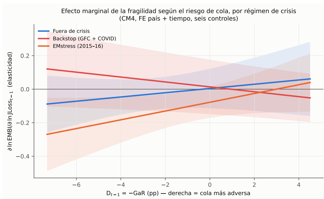
Figura 1.13: Elasticidad del spread a J\text{Loss}_{t-1} en función de D_{t-1} , por régimen (CM4 de la Tabla 1.9, efectos fijos de país y de tiempo, seis controles). Banda: IC 95 % (Driscoll–Kraay).
