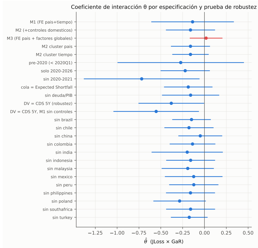
Figura 2.6: Coeficiente de interacción \theta por especificación y prueba de robustez; barras: IC 95 % (errores de Driscoll–Kraay). El punto estimado es negativo en la práctica totalidad de las filas —especificaciones, submuestras temporales y leave-one-country-out —, pero su intervalo de confianza cruza el cero en la mayoría de ellas sobre el panel completo.
