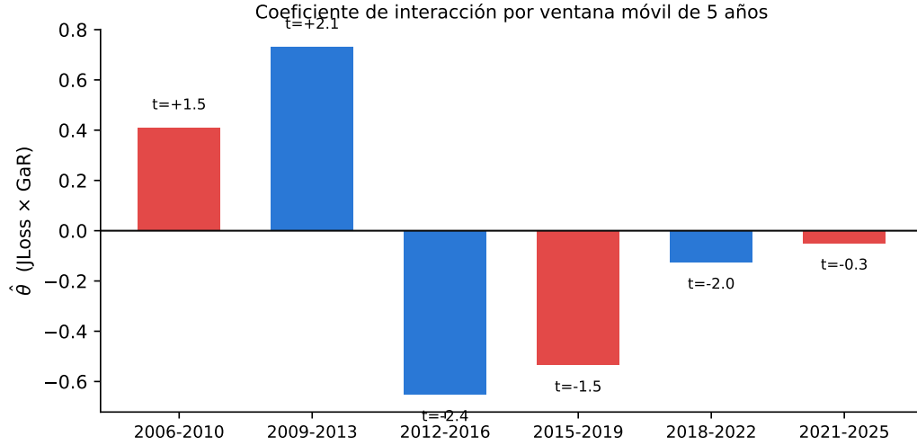
Figura 2.5: Coeficiente de interacción \theta ( JLoss \times GaR , especificación M2) estimado sobre ventanas móviles de cinco años, panel completo. Barras rojas: |t| < 1,64 .
