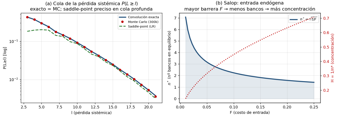
Figura 3.4: Robustez. (a) Validación de la cola de L : convolución exacta = Monte Carlo; punto de silla preciso en la cola profunda. (b) Salop: n^* = \sqrt{t/F} decreciente en la barrera de entrada.
