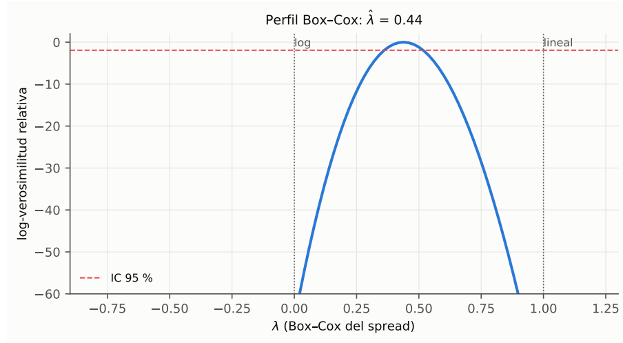
Figura 4.4: Log-verosimilitud concentrada de la transformación de Box–Cox del spread, con los regresores de la especificación principal y efectos fijos de país y de tiempo. Línea discontinua: umbral del IC 95 %.
