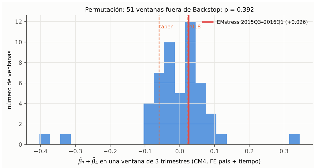
Figura 4.2: Distribución de \hat{\beta}_3 + \hat{\beta}_4 al reemplazar el episodio EMstress por cada ventana de tres trimestres consecutivos fuera de Backstop (CM4, efectos fijos de país y de tiempo, seis controles). Línea roja: 2015Q3–2016Q1; líneas discontinuas: taper tantrum y 2018.
