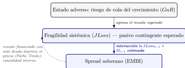
Figura 1.1: Mecanismo conceptual que resume los tres pilares del Capítulo 2: el riesgo de cola del crecimiento agrava el rescate bancario esperado, ese rescate esperado es la fragilidad sistémica JLoss , y el mercado la penaliza en el spread soberano. La flecha discontinua es la retroalimentación del spread hacia la fragilidad bancaria, que motiva rezagar los regresores. El tramo en azul es el que se estima.
