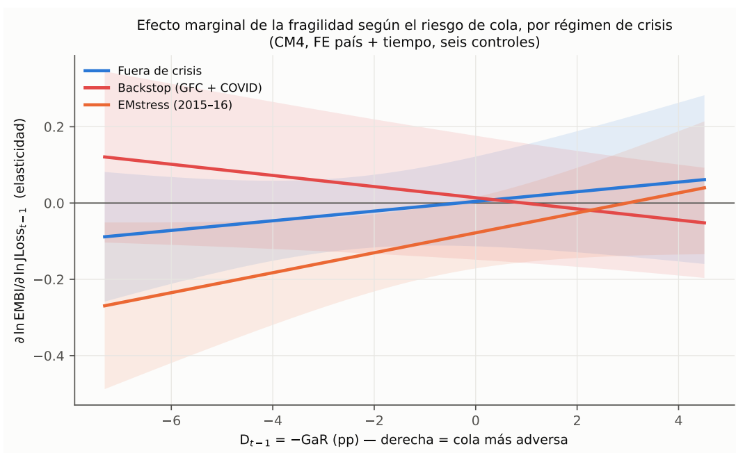
Figura 4.3: Elasticidad del spread a JLoss_{t-1} en función de D_{t-1} , por régimen (CM4 de la Tabla 4.5, efectos fijos de país y de tiempo, seis controles). Banda: IC 95 % (Driscoll–Kraay).
