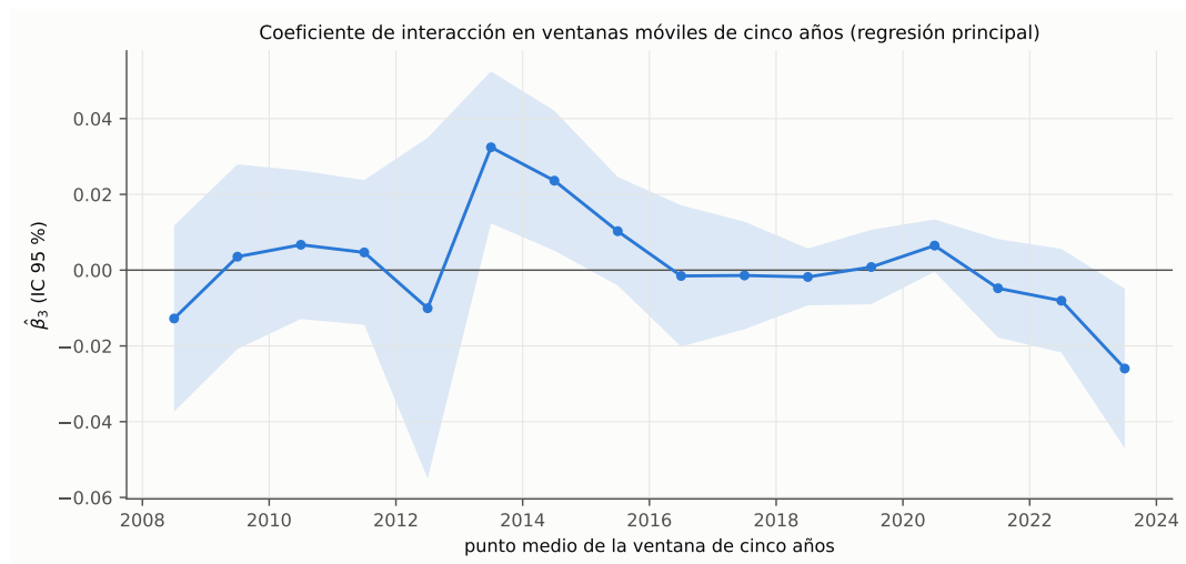
Figura 4.11: Coeficiente de interacción de la regresión principal en ventanas móviles de cinco años (IC 95 %). El eje horizontal marca el punto medio de la ventana.
