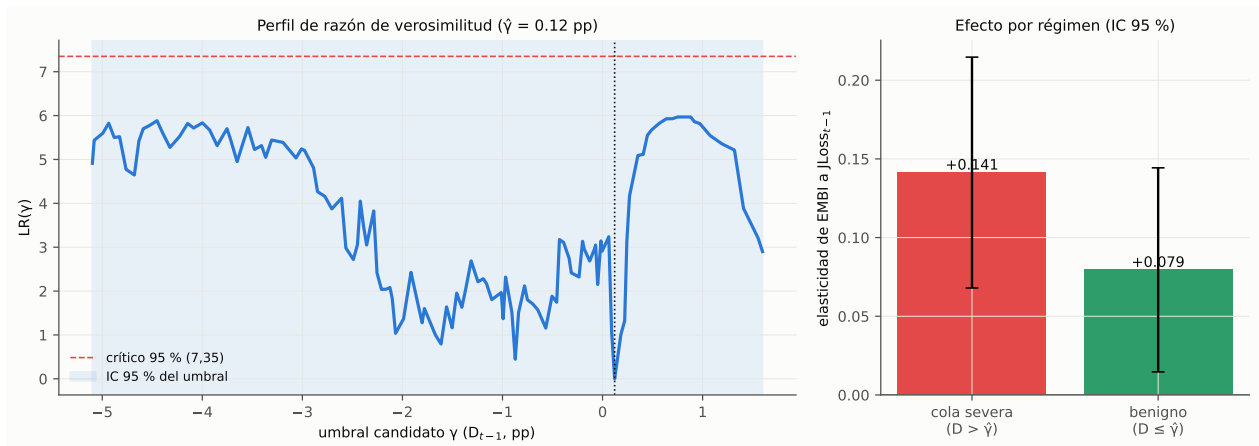
Figura 4.8: Modelo de umbral (Hansen, 2000) en logaritmos. Izquierda: perfil del estadístico LR(\gamma) , umbral estimado e IC 95 %. Derecha: elasticidad del spread a \text{JLoss}_{t-1} en cada régimen (IC 95 %, Driscoll–Kraay).
