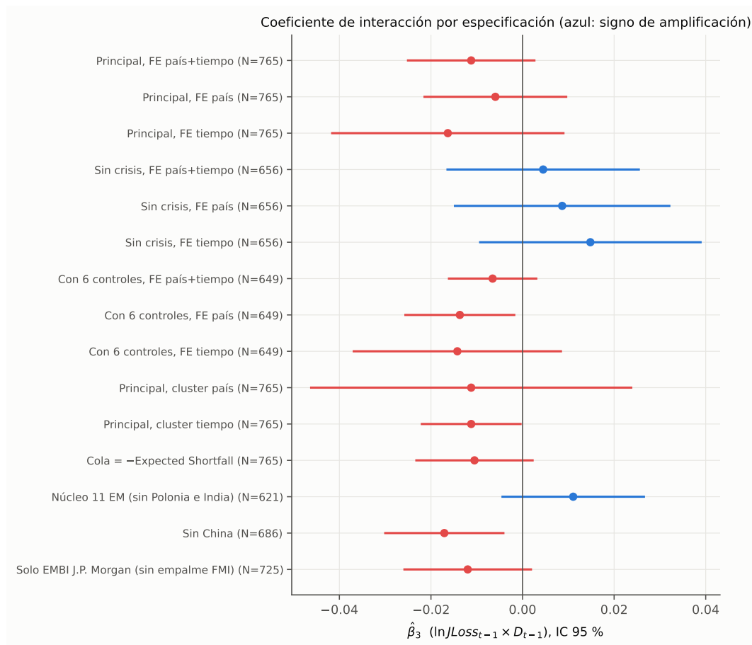
Figura 4.9: Coeficiente de interacción \hat{\beta}_3 por especificación, con IC 95 % (Driscoll–Kraay salvo indicación). Azul: signo de amplificación; rojo: signo opuesto.
