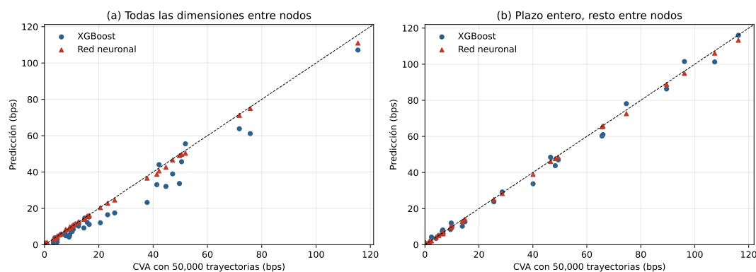
Figura 9: Predicción frente a CVA con 50,000 trayectorias en valores entre los nodos de la parrilla, dentro de los rangos de entrenamiento: (a) todas las dimensiones entre nodos; (b) plazo entero y el resto entre nodos.
